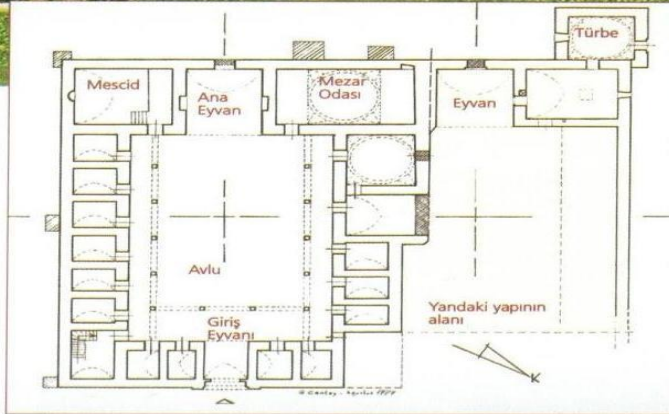
Darüşşifa'nın zemin kat planı (G. Cantay) / Entrance floor plan of the darüşşifa
